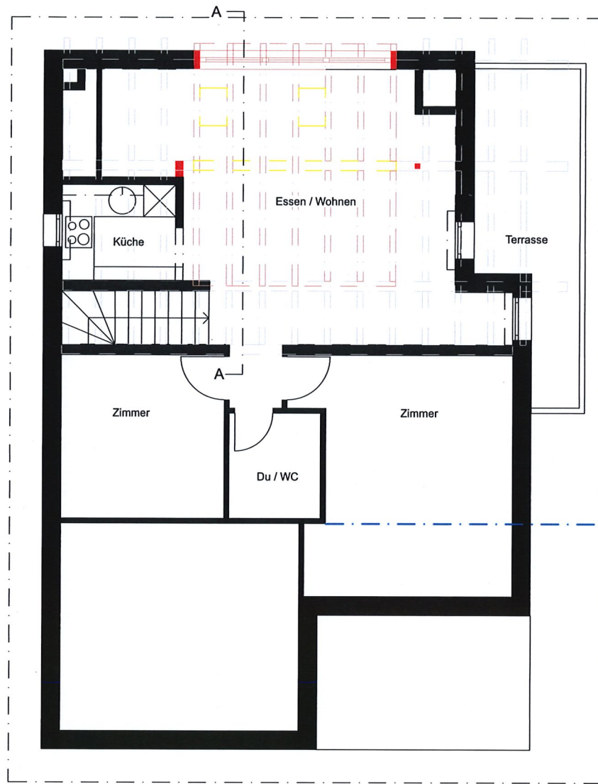
Dachgeschoss - Projekt
